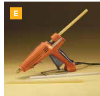
3M™ Schmelzklebstoff-Auftragsgerät AE II. Niedriges Volumen.
