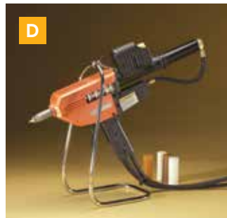
3M™ Heißschmelzkleber-Druckluftpistole PG II mit Speedloader. Hohes Volumen.
