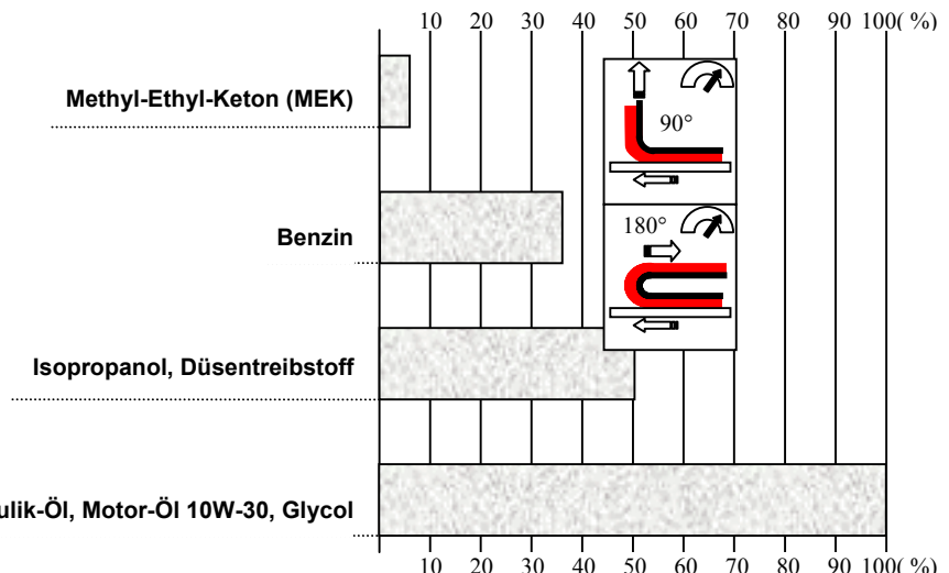
Diagramm 2: Lösemittelbeständigkeiten VHB™ Klebebänder
