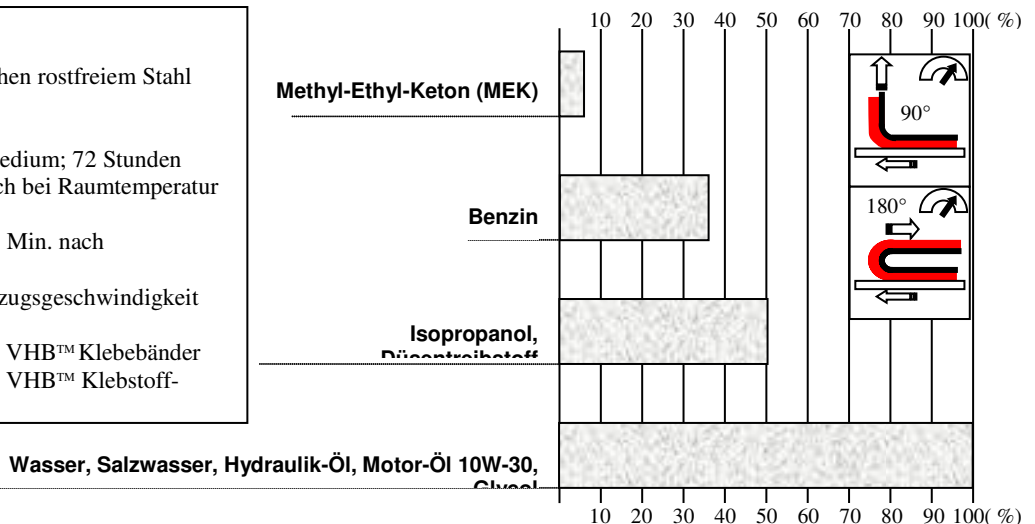
Diagramm 2: Lösemittelbeständigkeiten VHB™
